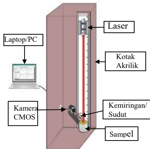
Gambar 2. Desain sistem alat identifikasi pupuk oplosan,
