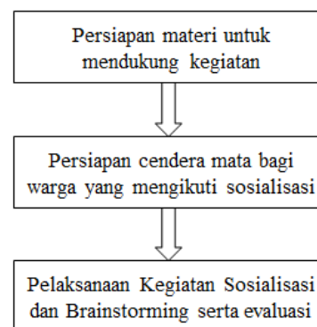
Gambar 1. Tahapan Penelitian
