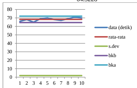
Gambar 3 Grafik Uji Keseragaman Data Proses Pengelasan
