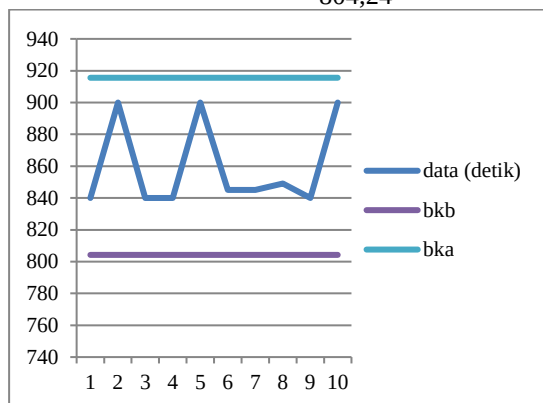
Gambar 5 Grafik Uji Keseragaman Data Proses Perakitan
