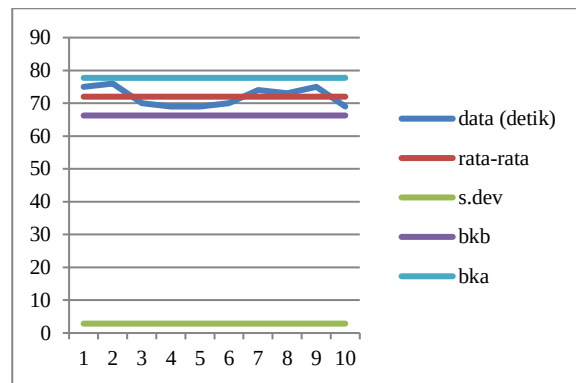
Gambar 6 Grafik Uji Keseragaman Data Proses Pendempulan
