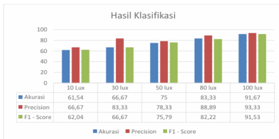
Gambar 4. Diagram Hasil Klasifikasi Menggunakan Metode K-NN
